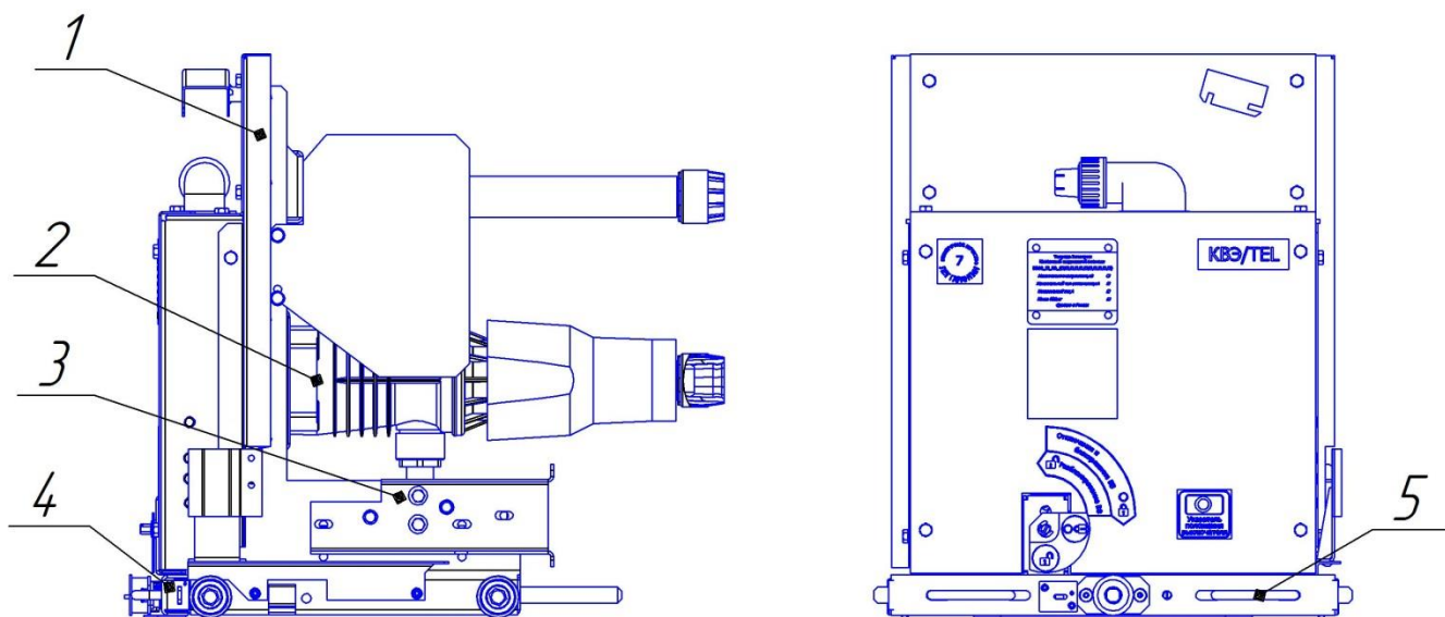
а) кассетный выкатной элемент KBЭ до 1250 А
